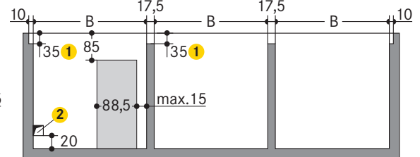
Reihenanlage
