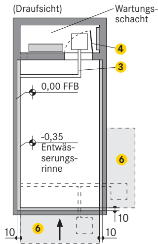
(Draufsicht)
