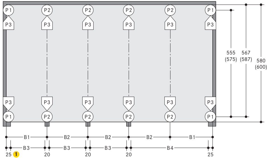
Grundriss
