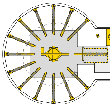
Schnitt Einfahrtsebene
