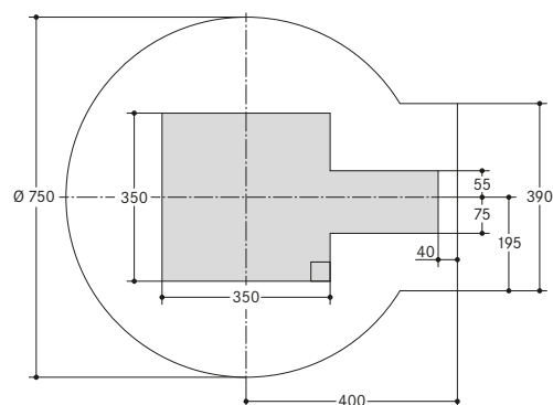
Fundament Draufsicht
