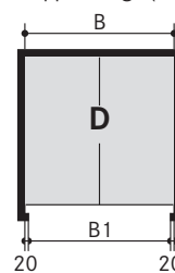
Doppelanlage (6 Pkw)
