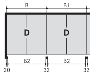
Reihengarage mit Doppeltoren (je 6 Pkw)
