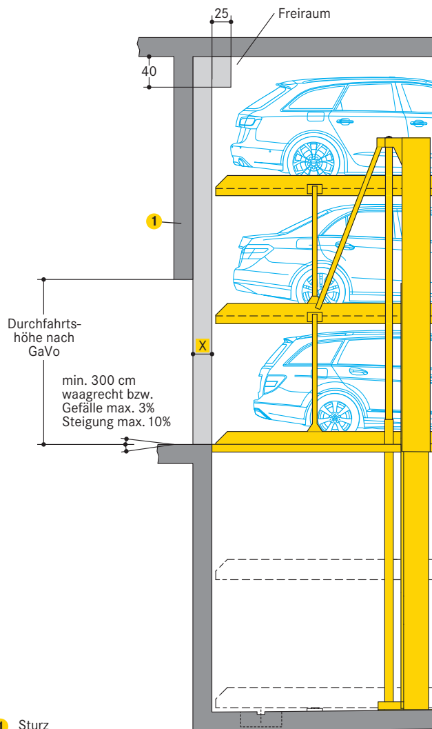
Einzelanlage (3 Pkw)
